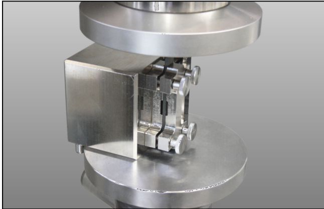
Druckvorrichtungen (End loading) zwischen zwei Druckplatten, zur Messung des Druckmoduls
